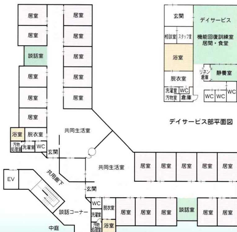
ユニット部平面図
